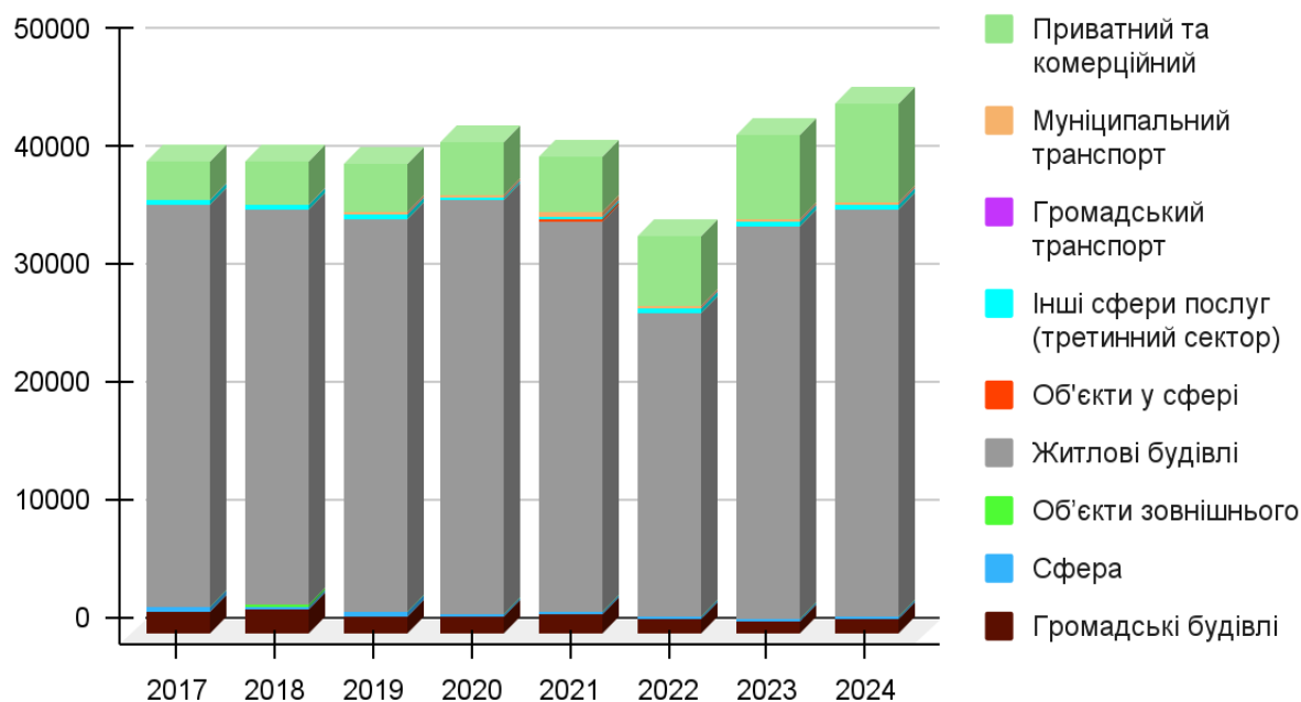
Малюнок 2.15. Зведений енергетичний баланс за період 2017-2024 роки за категоріями кінцевих споживачів
