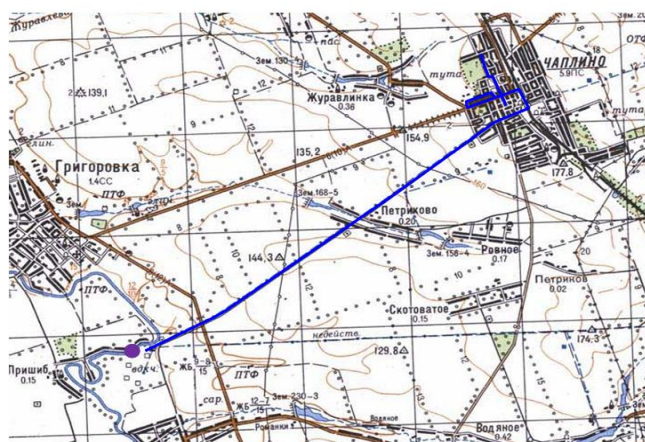
Схема мережі централізованого водопостачання селища Чаплине Дубовиківської громади Синельниківського району Дніпропетровської області
