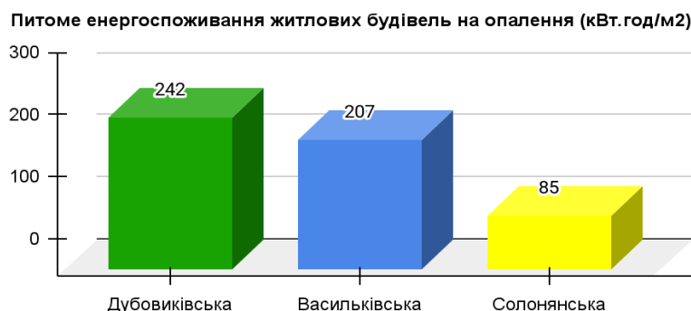
Малюнок 2.22. Питоме енергоспоживання житлових будівель на опалення (кВт·год/м²)
