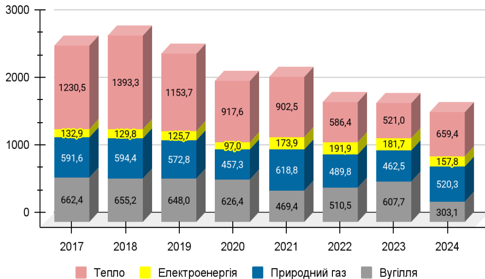
Малюнок 2.1. Обсяги споживання енергоресурсів в громадських будівлях Дубовиківської територіальної громади, МВт.год
