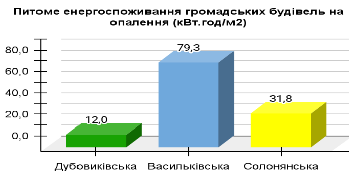
Малюнок 2.21. Питоме енергоспоживання громадських будівель на опалення (кВт·год/м²)
