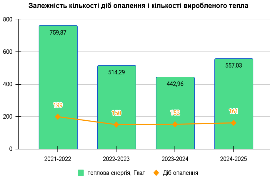
Малюнок Д2.15. Залежність кількості діб опалення і кількості виробленого тепла
